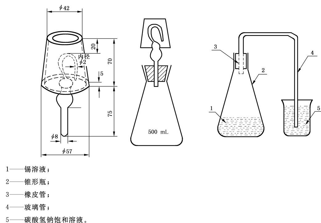
图 1 锡还原装置示意图
